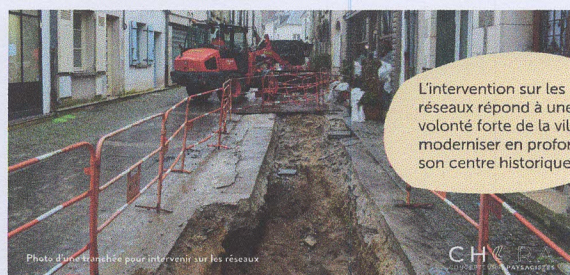
Photo d'une tranchée pour intervenir sur les réseaux
